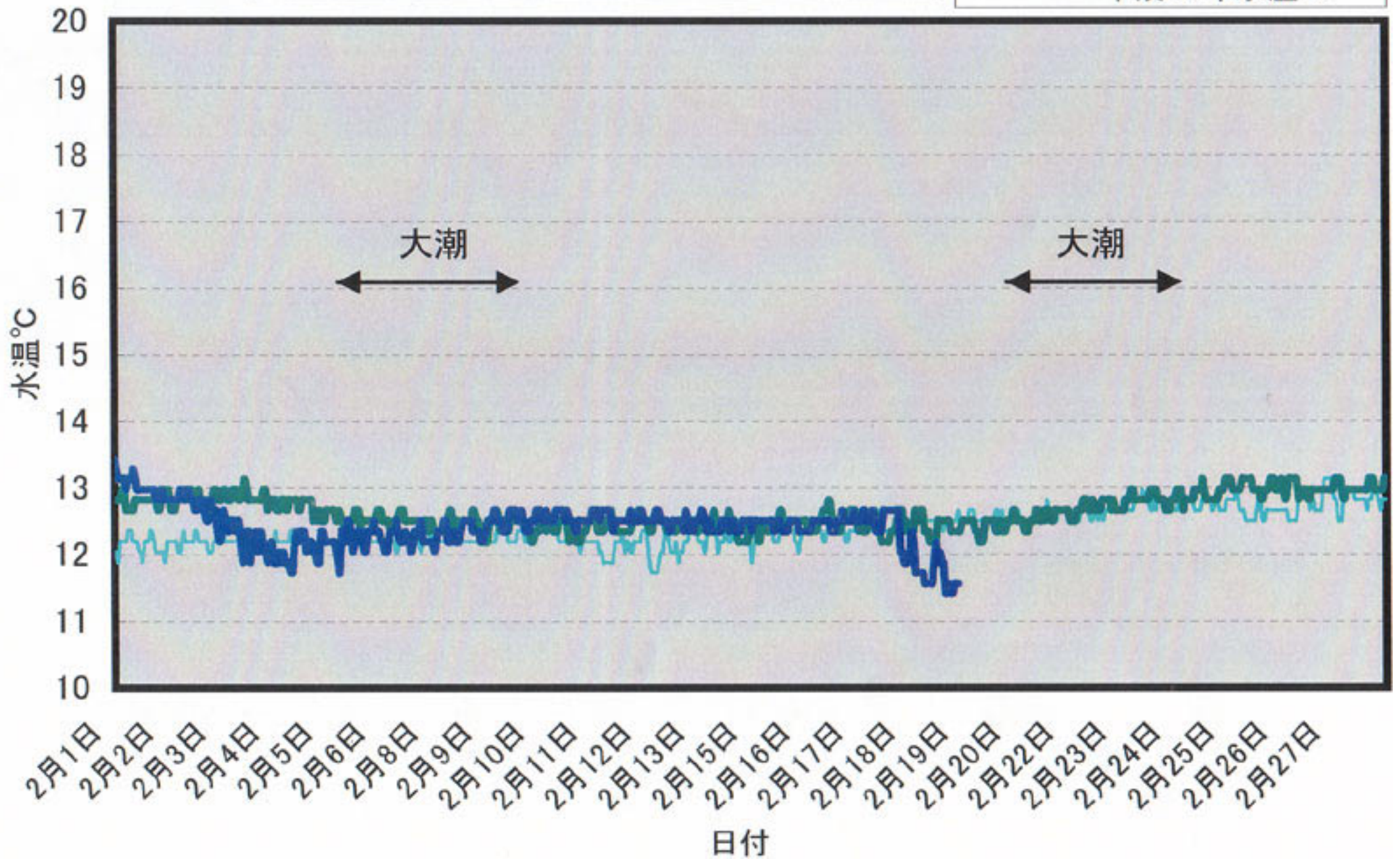
2月 天草竜ヶ岳地区1時間毎の水溫変化(5m層)
